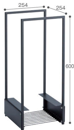
下部スペースに荷造り紐などを収納可能。
