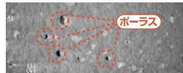
鏡面仕上げセラミックタイル表面（100倍）
